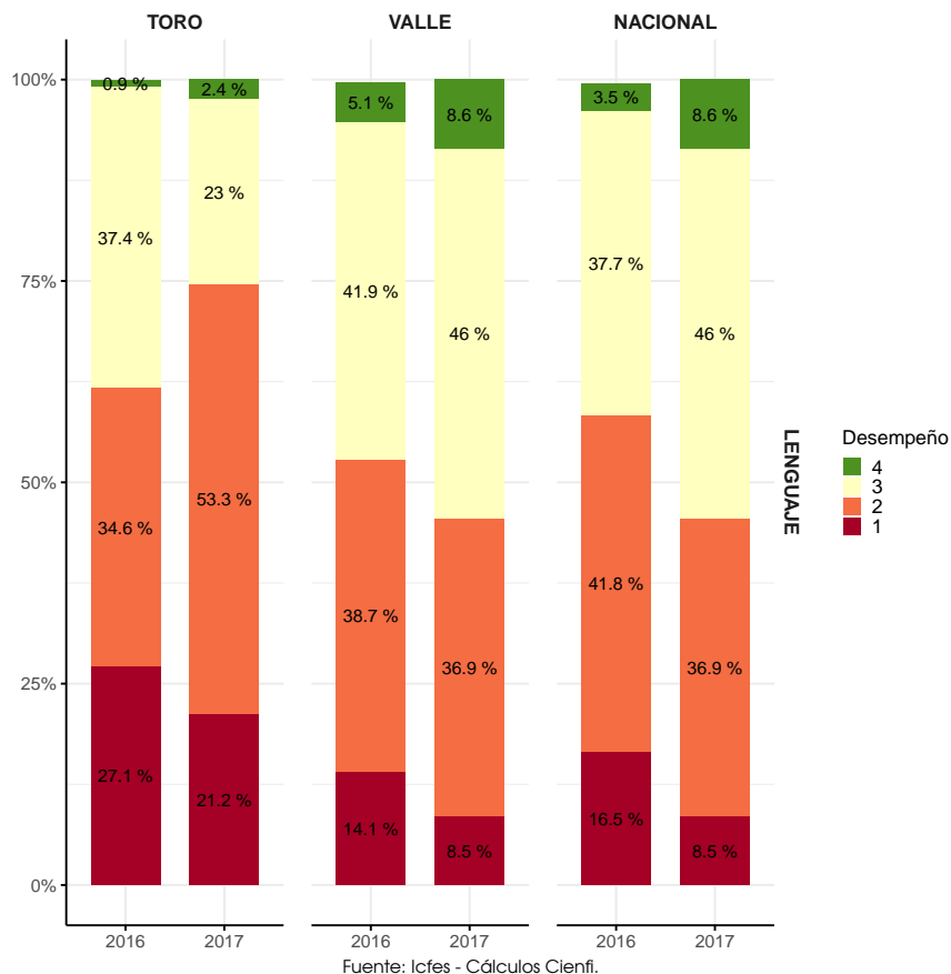
Figura 6.4: Evolución de la distribución de desempeño de los estudiantes en Toro para la competencia de Lenguaje en Saber 9
