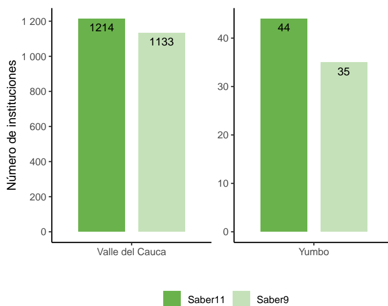
Figura 3.6: Número de colegios con estudiantes tomando el examen Saber 9 2017 y número de colegios con estudiantes tomando el examen Saber 11 2019 en Valle del Cauca y Yumbo)
